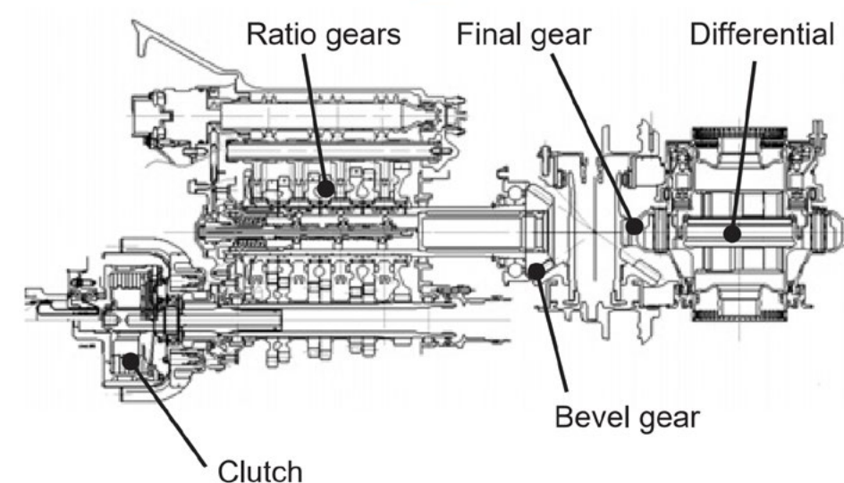
Fig. 2 Structure of F1 gearbox internals
