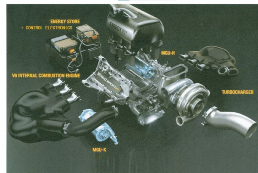
Fig. 4. F1 Power Unit components – 2014 [Renault]
