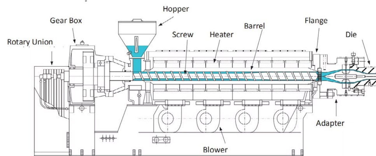
شمایی از دستگاه اکسترودر
