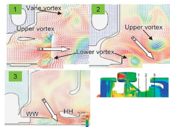
Fig. 15 BBD vortices
