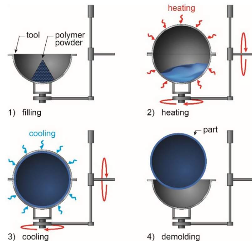
شمایی از فرایند قالب‌گیری چرخشی
