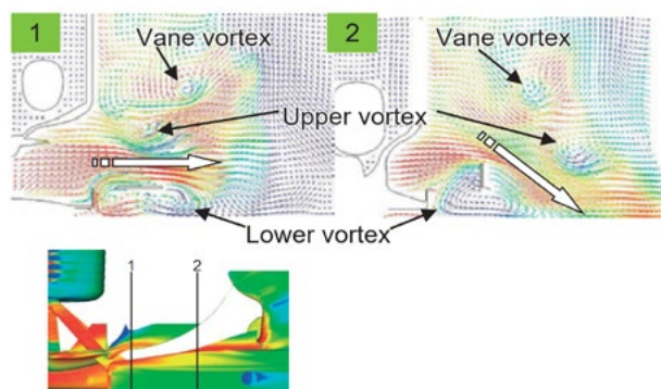
Fig. 19 ONF vortices
