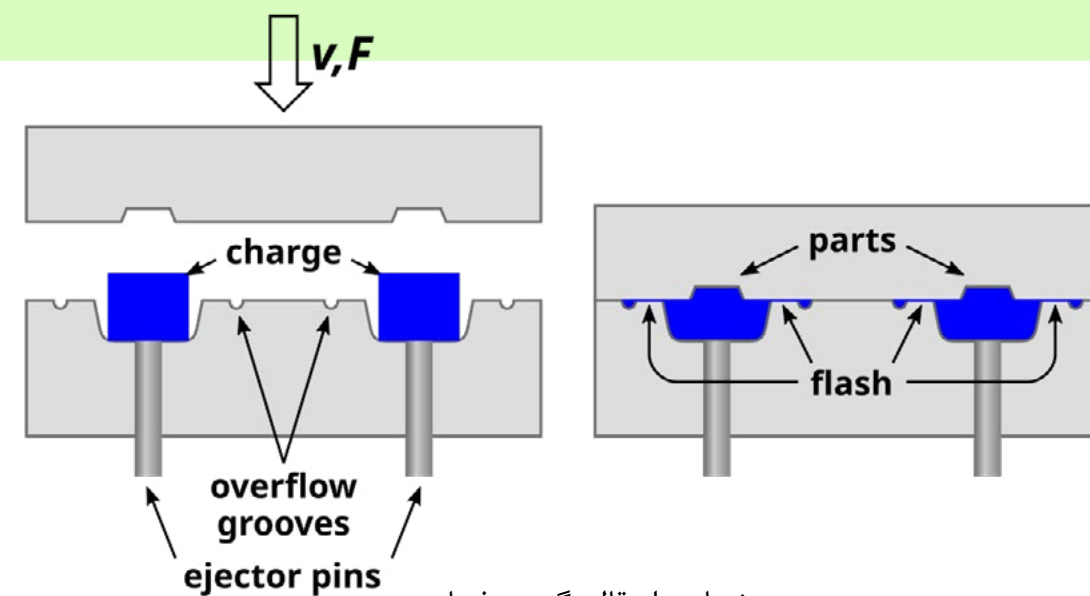
شمایی از قالب‌گیری فشاری
