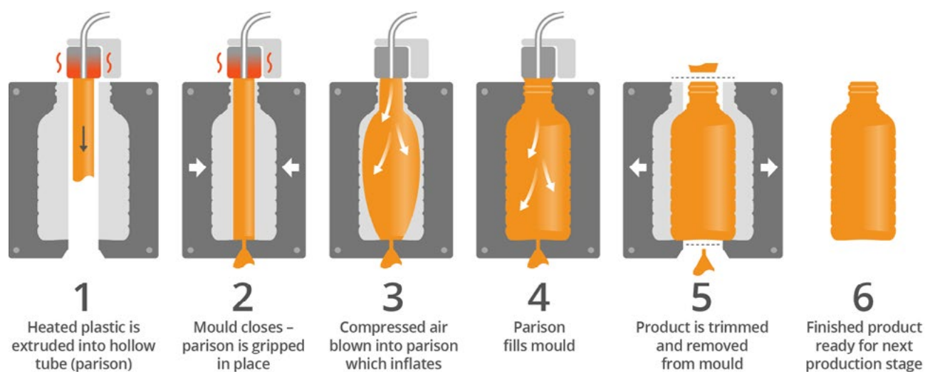
شمایی از فرایند قالب گیری دمشی
