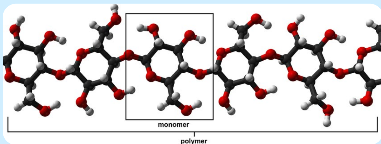
نمایی از ساختار مونومر و پلیمر
